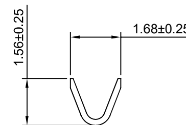
SEC:B-B
