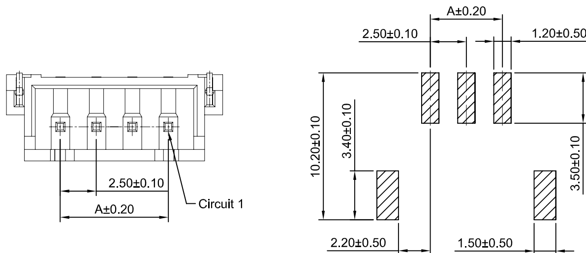
P.C.B LAYOUT
