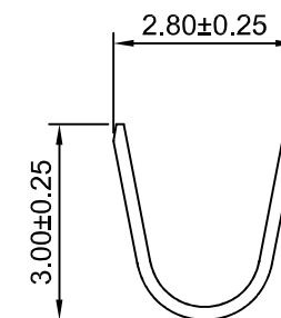
SEC:A-A
